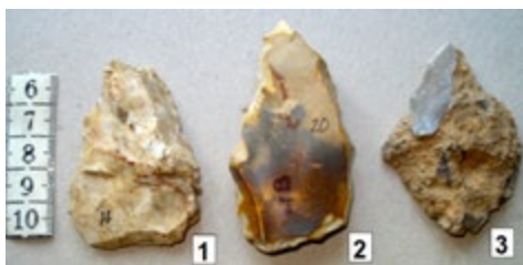
Obr. 10. Střední paleolit. Libhošť – U silnice 1 a 2. 1 – 3 mousterské hroty
